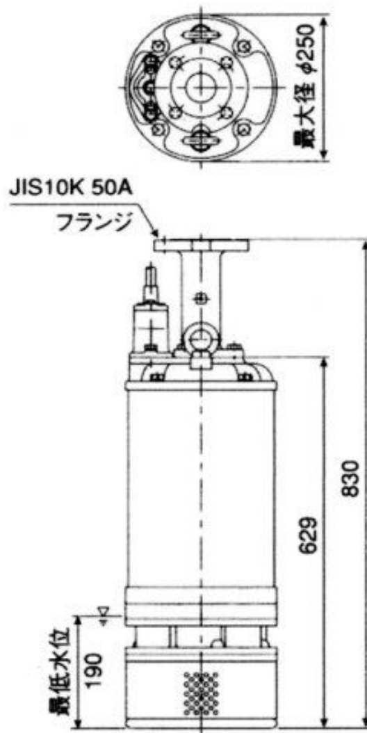
【外形寸法図】
